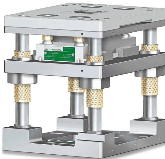
复合模
