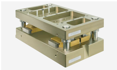
完整工具
