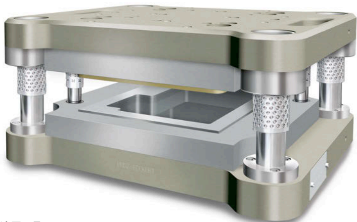
全冲压工具
